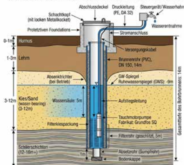
Schema eines 14 m tiefen Bohrbrunnens mit 5 m Wassersäule
