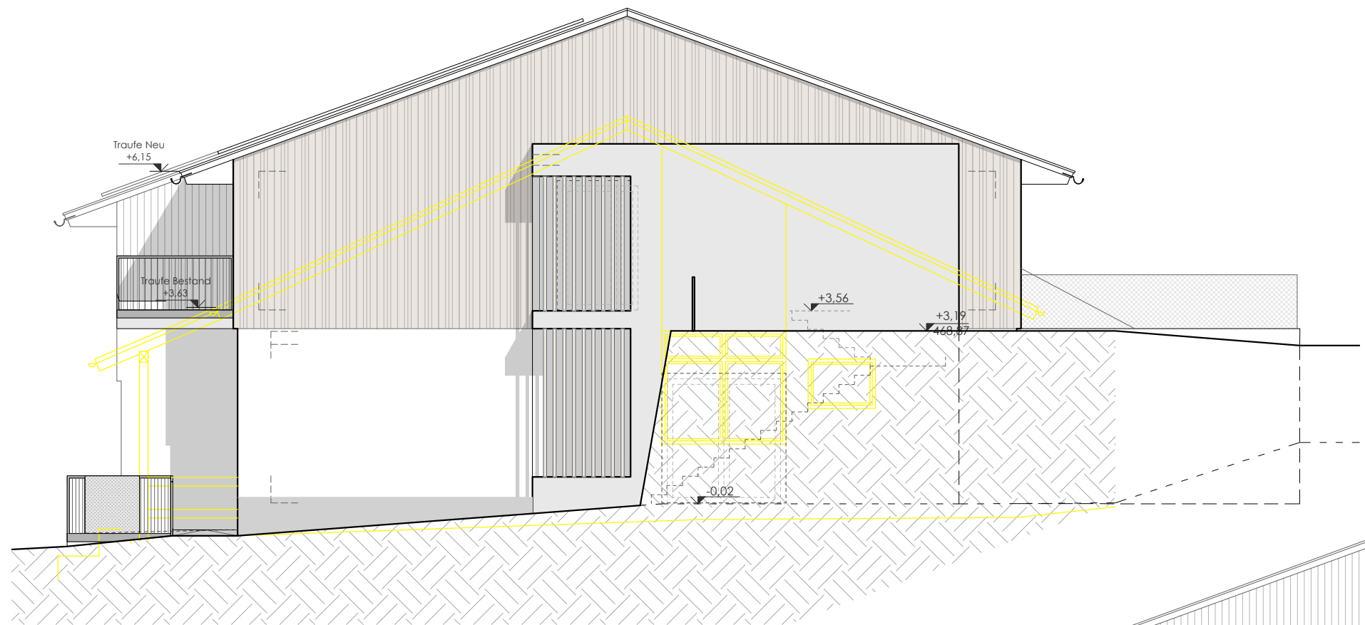
ANSICHT OST
