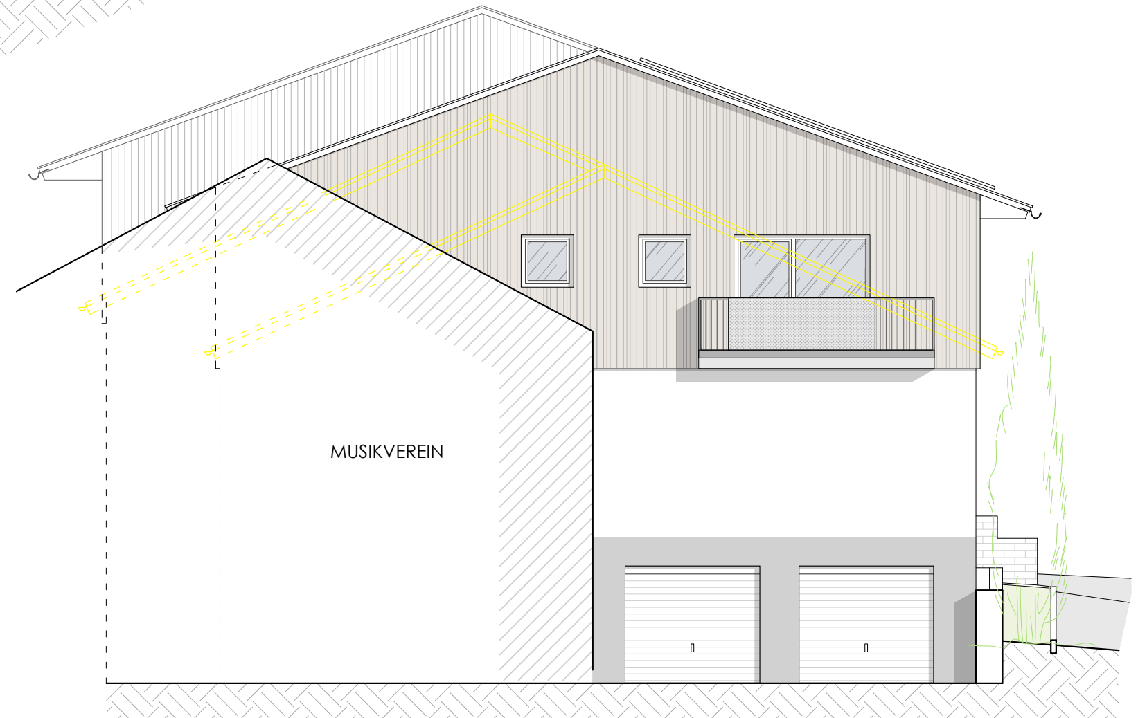
ANSICHT WEST
