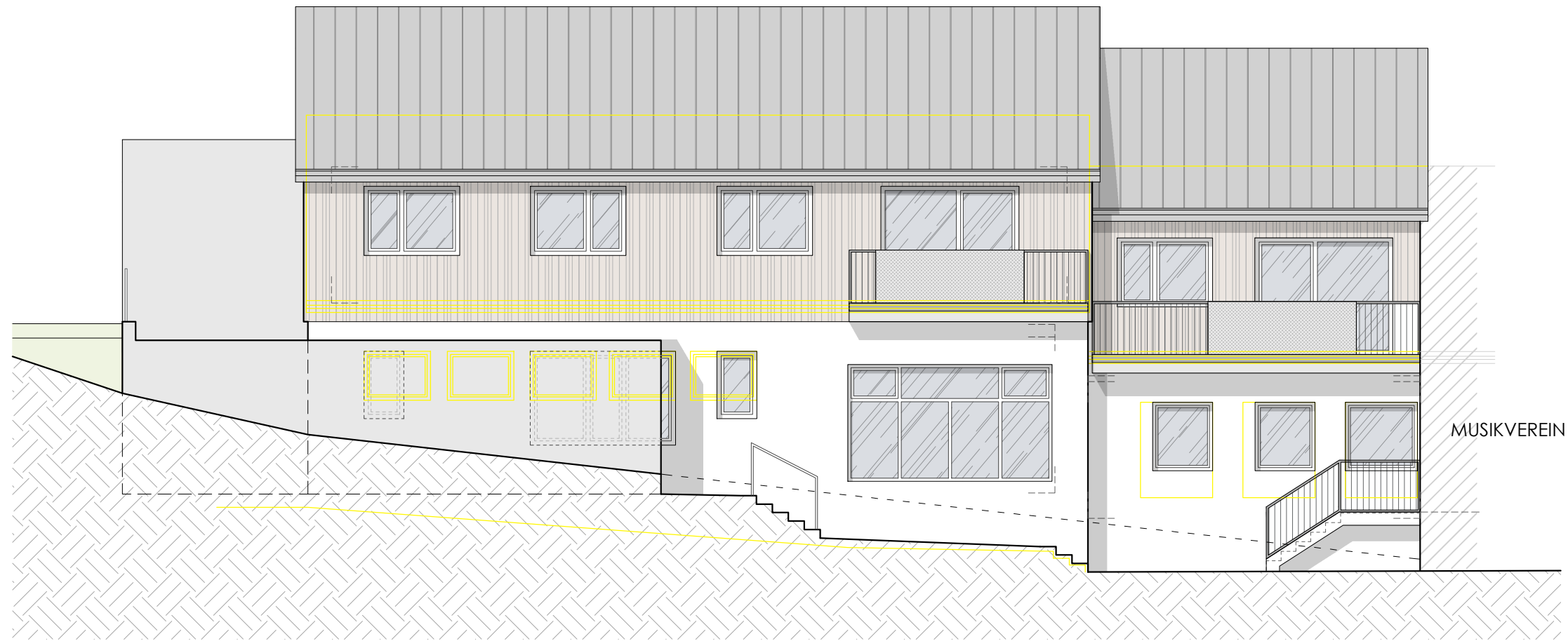
ANSICHT NORD
