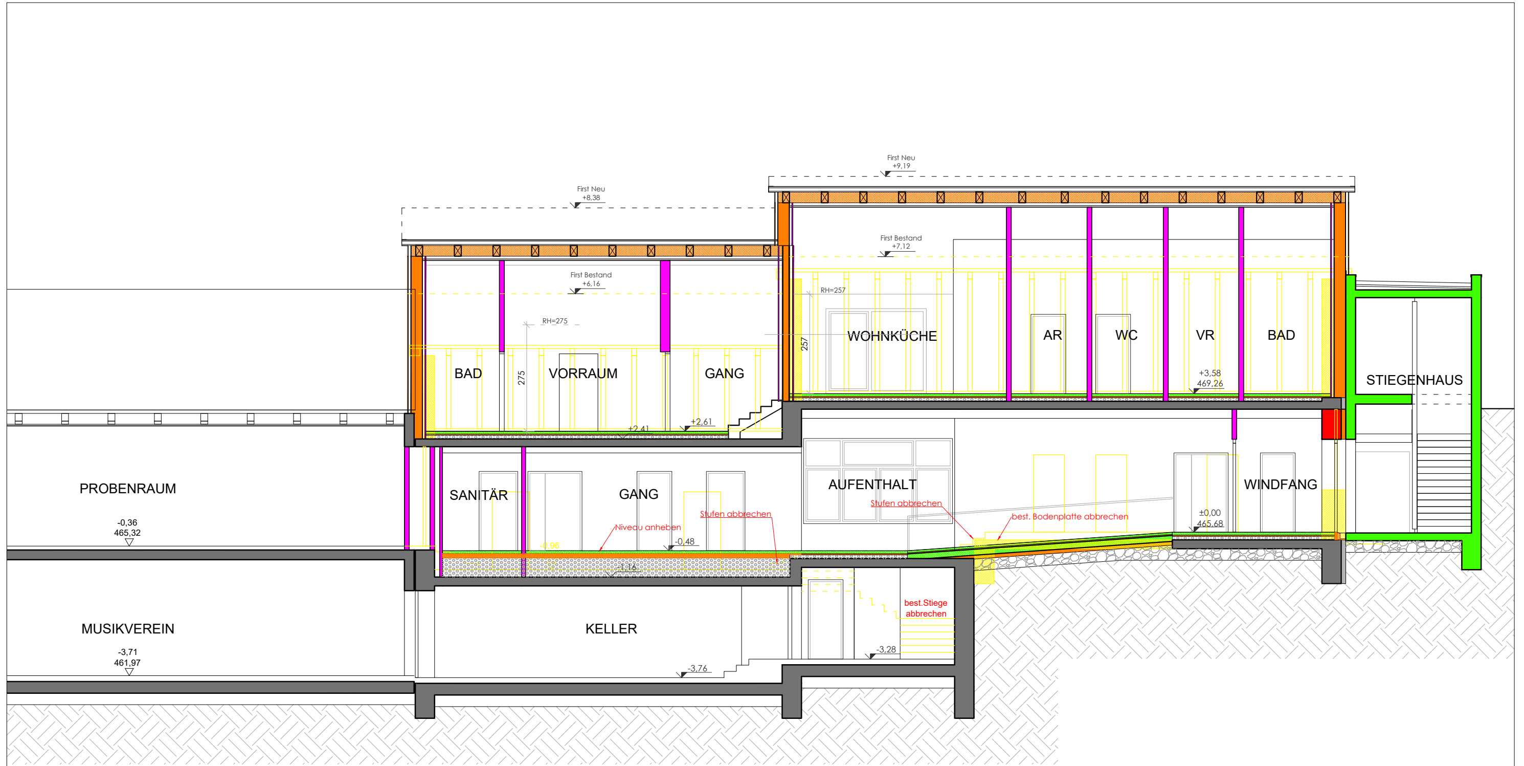
SCHNITT B-B
