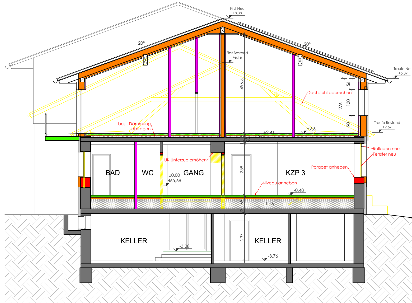
SCHNITT A-A
